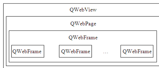
Gambar 4 Skema Hubungan Antarclass Webkit (Sumber: Kurniawan, 2011)
