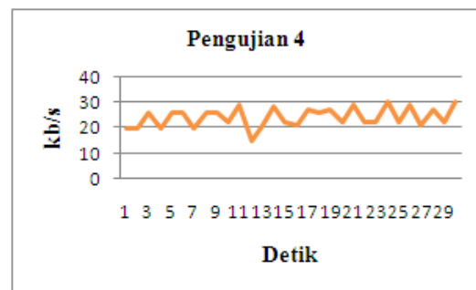
Gambar 18 Grafik Pengujian 4 (Besar Data tiap Detik) Webcam 5 MP
