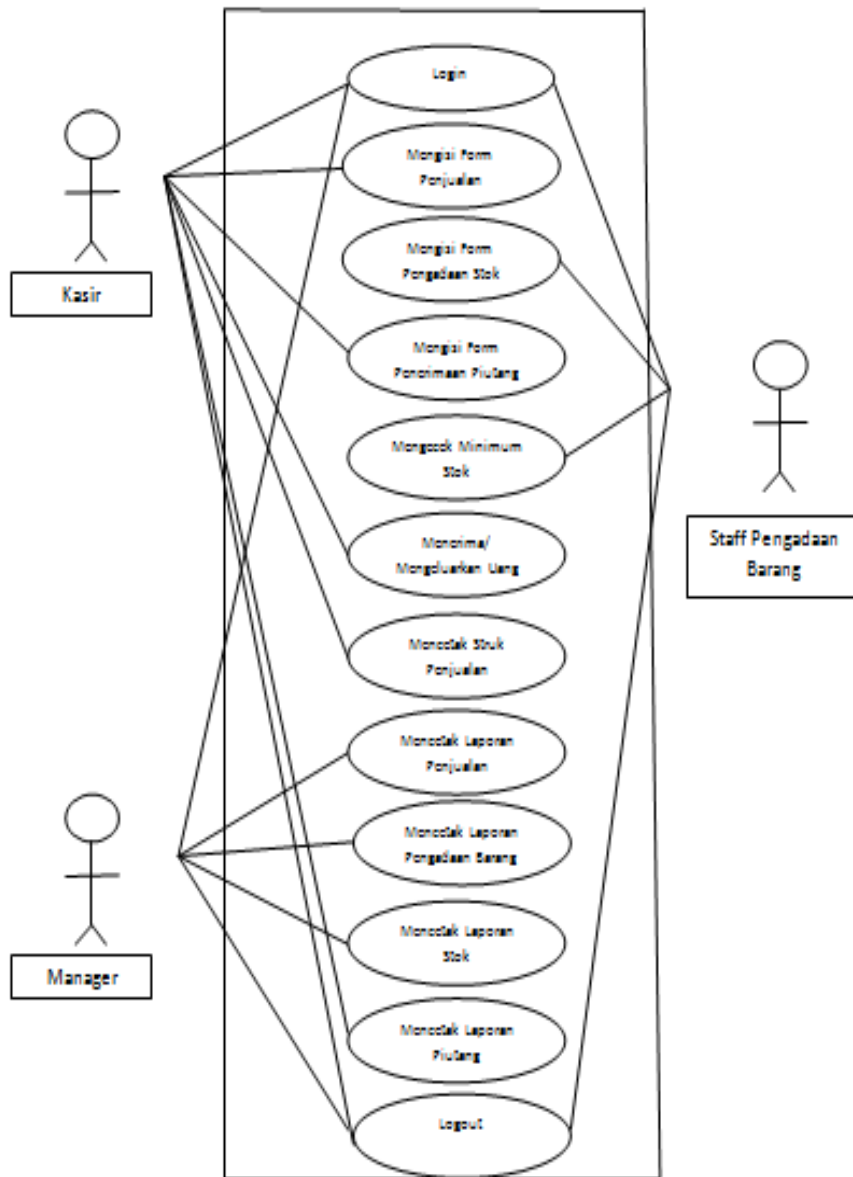
Gambar 2 Use Case Diagram Sistem Informasi Penjualan yang Diusulkan
